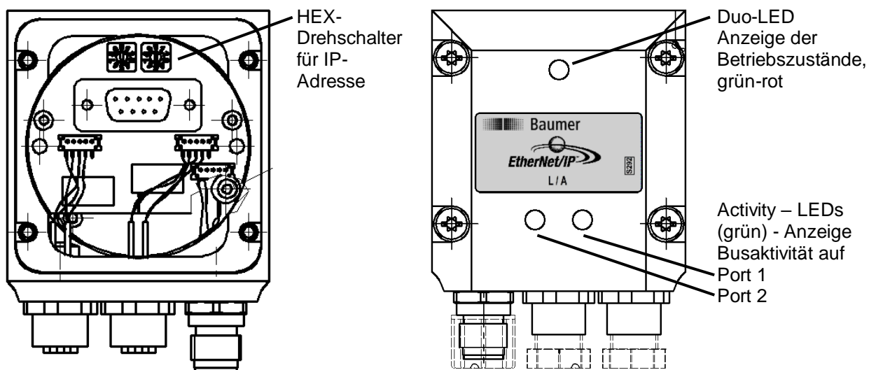
Bild 4: Bushaube – Elektrische Anschlüsse und LEDs
