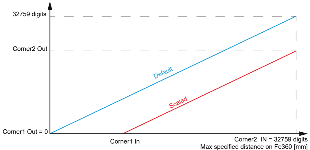
Abb. 24: Skalierung – Fixed Slope Gradient, Teach Corner 1
