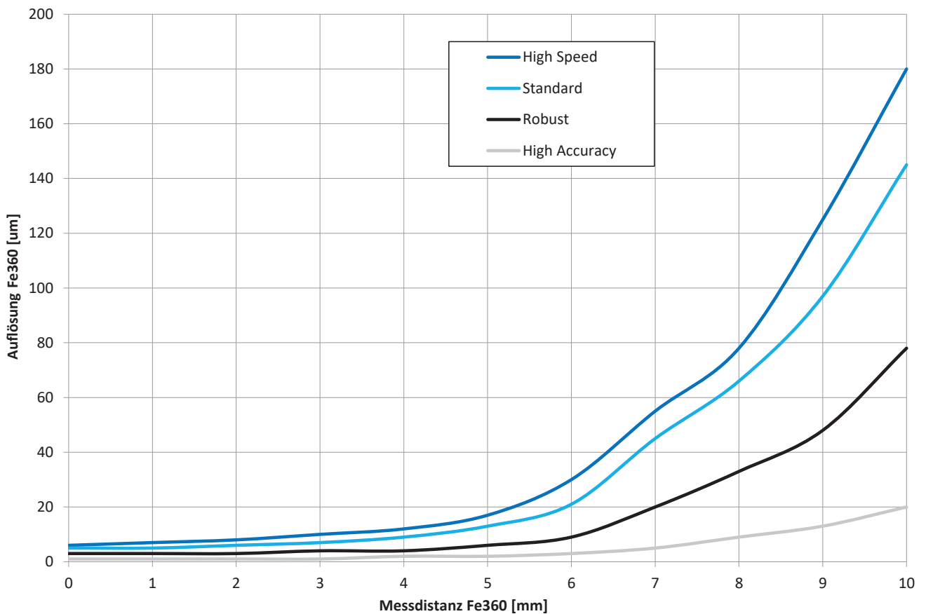
Abb. 22: Einfluss des Filters auf die Auflösung
