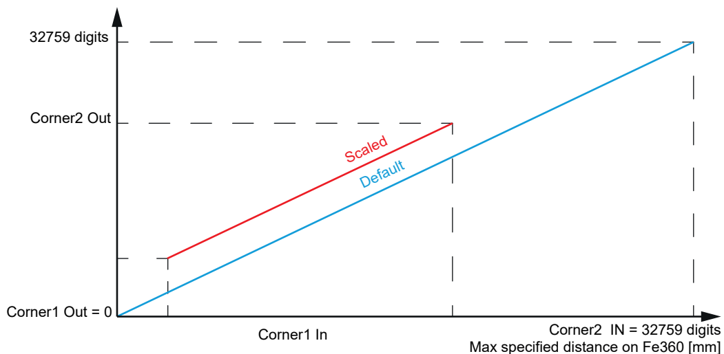
Abb. 23: Skalierung – In vs out
