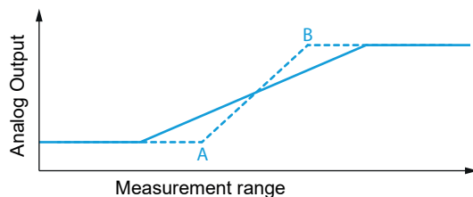
Abb. 19: Reduzierter Bereich des Analogausgangs Wertes für verbesserte Genauigkeit (Analogwert erhöht sich mit der Entfernung)
