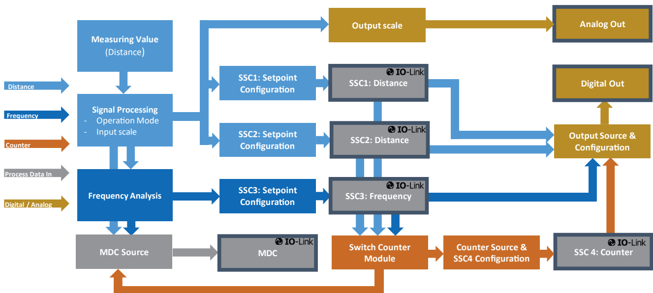
Abb. 21: Signalverarbeitungskette (schematische Darstellung)
