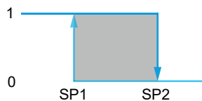
Abb. 5: Sensor im Messmodus Two Point
