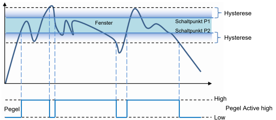
Abb. 11: Verhalten des Schaltausgangs bei Modus Window und negativer Hysterese ( Right Aligned )
