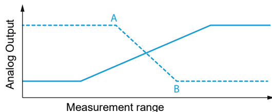
Abb. 20: Reduzierter und invertierter Bereich des analogen Ausgangswertes für verbesserte Genauigkeit und unterschiedliche Steigung (Analogwert nimmt mit der Entfernung ab)
