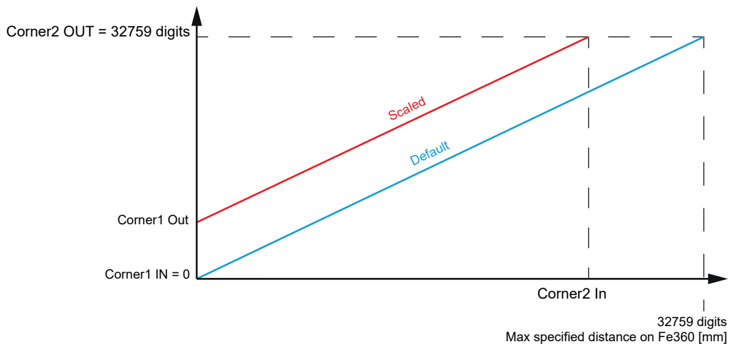
Abb. 25: Skalierung – Fixed Slope Gradient, Teach Corner 2
