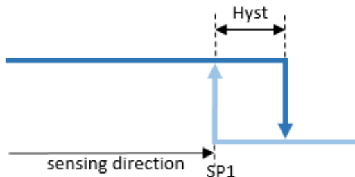
Abb. 7: Darstellung Hysterese
