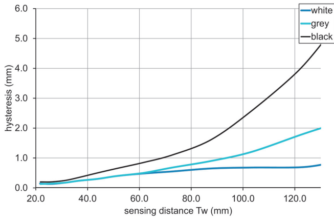
迟滞曲线
