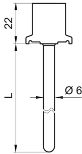
Tri-Clamp Ø 25 (BCID: C01) 3-A
